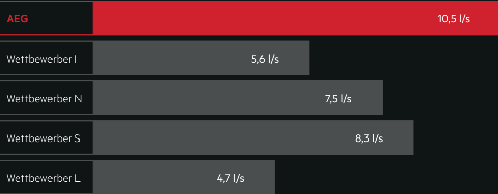
SAUGLEISTUNG / LUFTSTROM*
